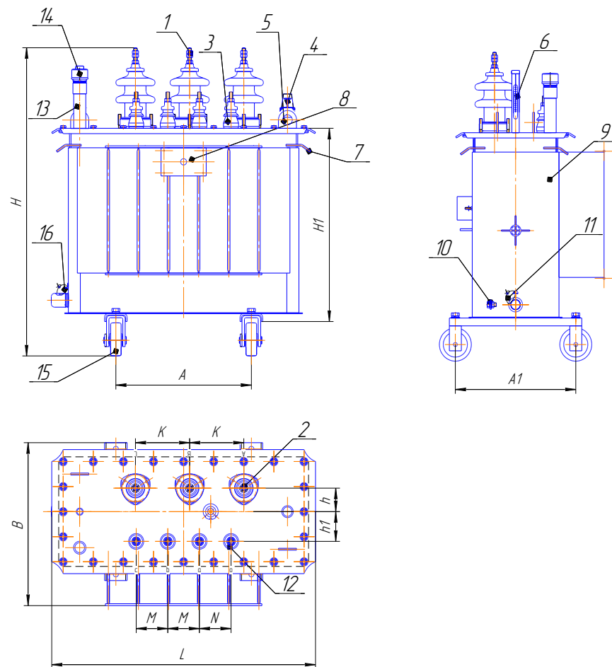
Общий вид трансформаторов ТМГ-63
