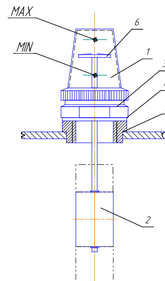
1 – прозрачный колпак; 2 –поплавок; 3 – корпус; 4 – прокладка; 5 – втулка на крышке; 6 –сигнальный шток
